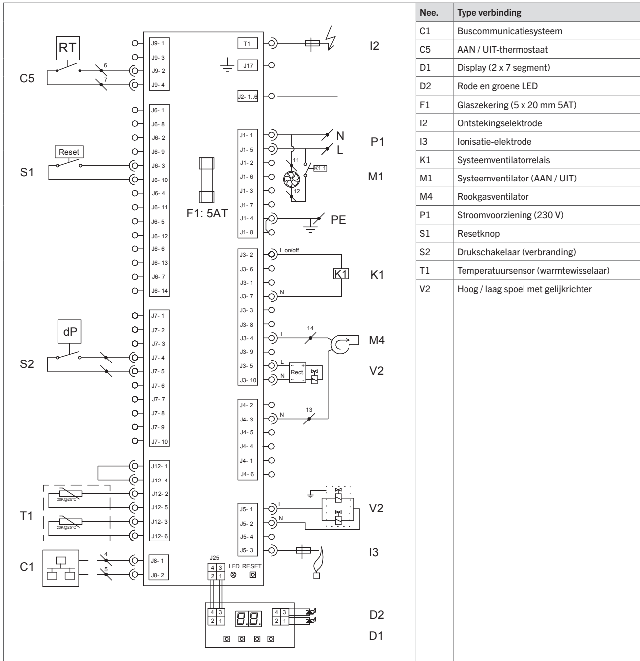
Figuur 12 - Elektrisch schema
