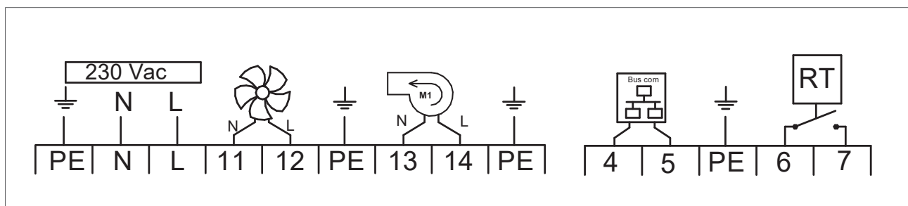
Figuur 13 - Hoofdaansluitingen voor de installatie
