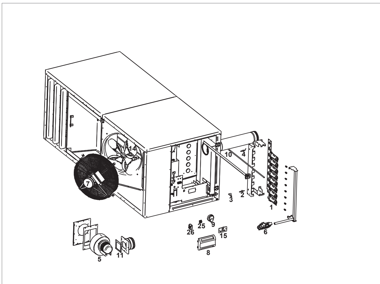
Figuur 14 - Exploded view van de DXE
