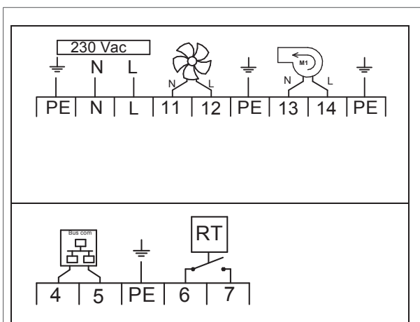
Figuur 3 - De verbindingsklemmen van de luchtverwarmer
